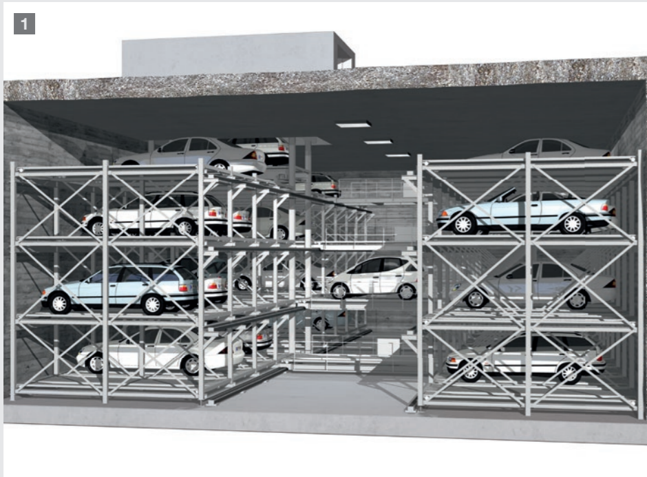
1 MasterVario LS transportiert Fahrzeuge per Lift zur Parkebene und mit Shuttle zum Stellplatz
